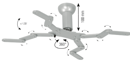
Projektorhalterung Basic II
